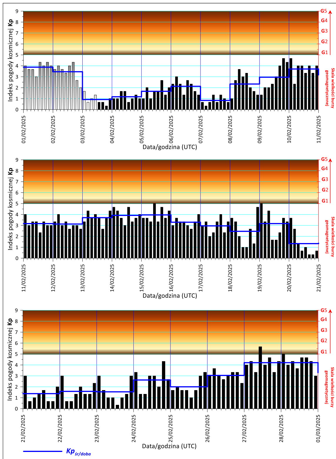
Rys. 2. Zmiany indeksu Kp „pogody kosmicznej” w miesiącu lutym 2025 r (dane wg. NOAA).
