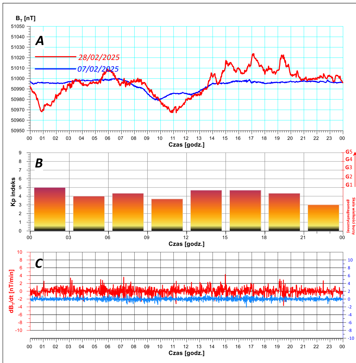
Rys. 4. Magnetogram z monitoringu modułu całkowitego wektora indukcji pola geomagnetycznego zarejestrowany w dniu 28/02/2025 r. na stacji geodynamicznej PSG zlokalizowanej w Hołownie (gm. Podedworze, pow. parczewski).
