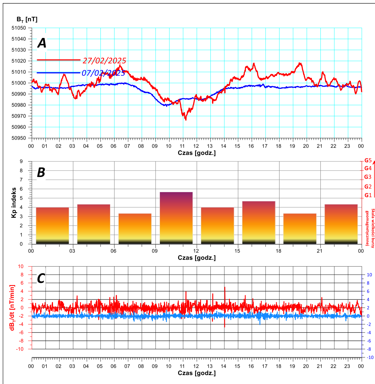
Rys. 3. Magnetogram z monitoringu modułu całkowitego wektora indukcji pola geomagnetycznego zarejestrowany w dniu 27/02/2025 r. na stacji geodynamicznej PSG zlokalizowanej w Hołownie (gm. Podedworze, pow. parczewski).
